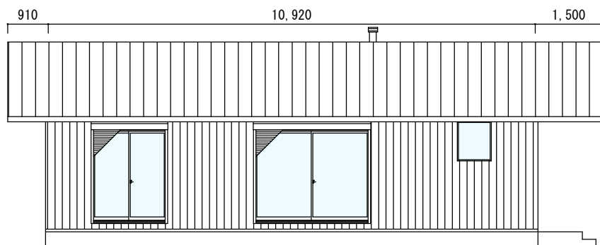
南面 立面図
